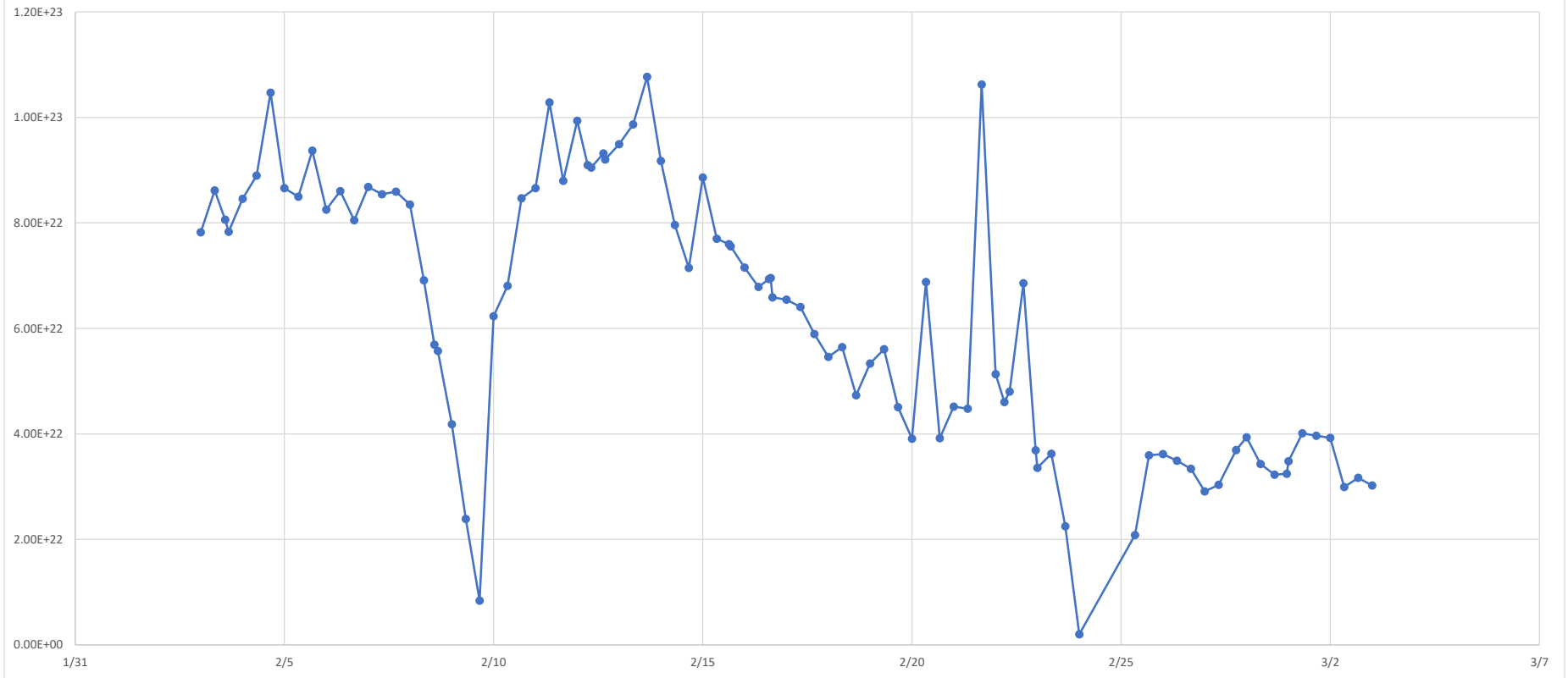
NOAA 11967 -> AR 11990
